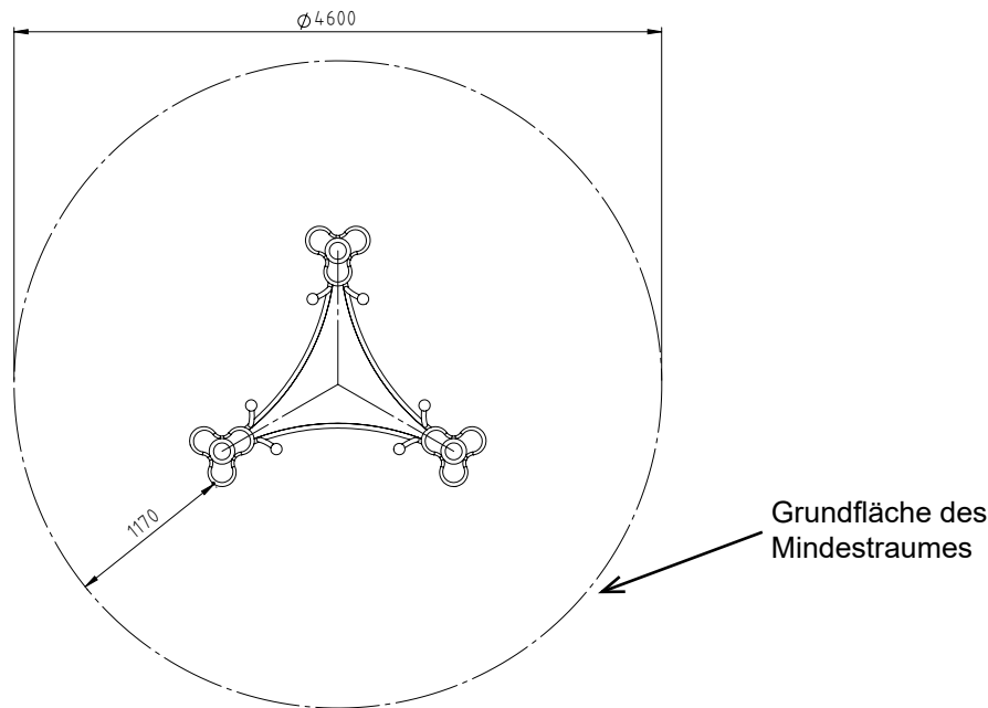
Skizze 3: Draufsicht
