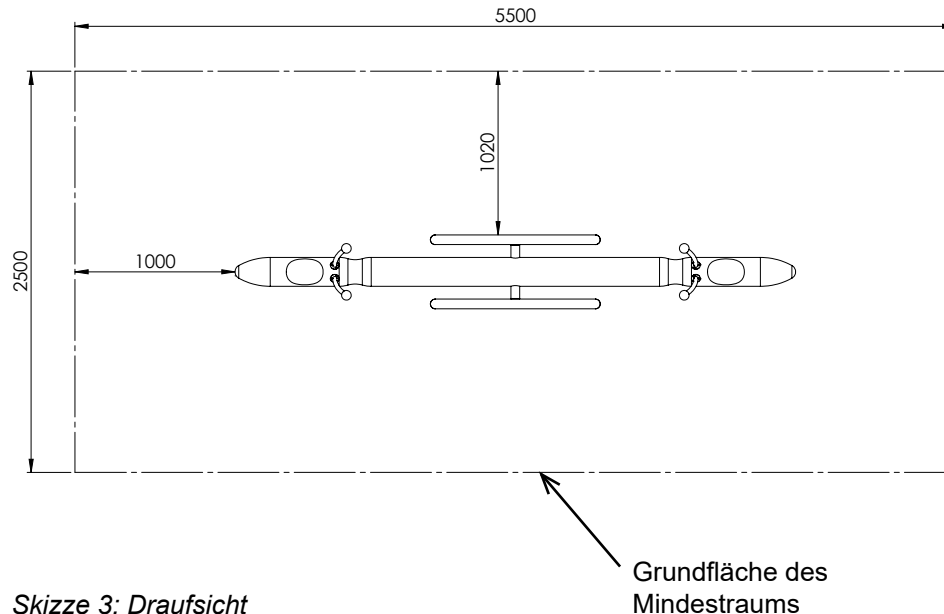
Skizze 3: Draufsicht
