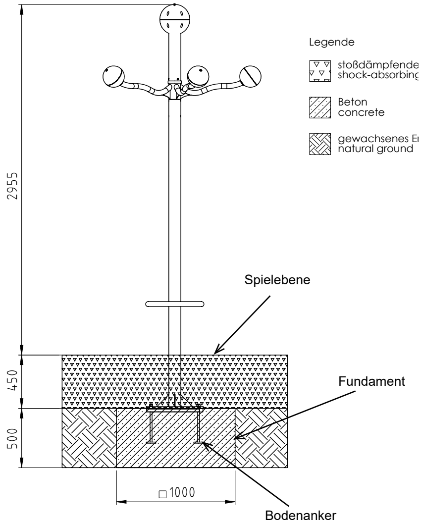
Skizze 2: Fundamentplan
