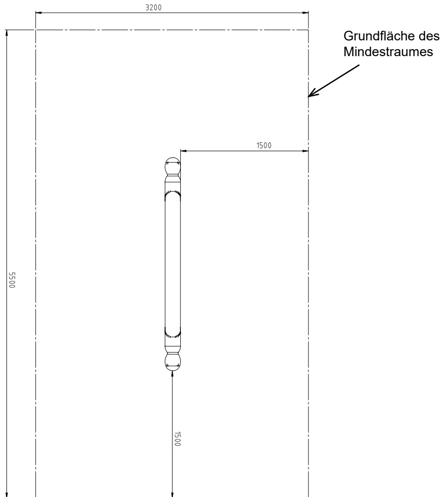
Skizze 3: Draufsicht
