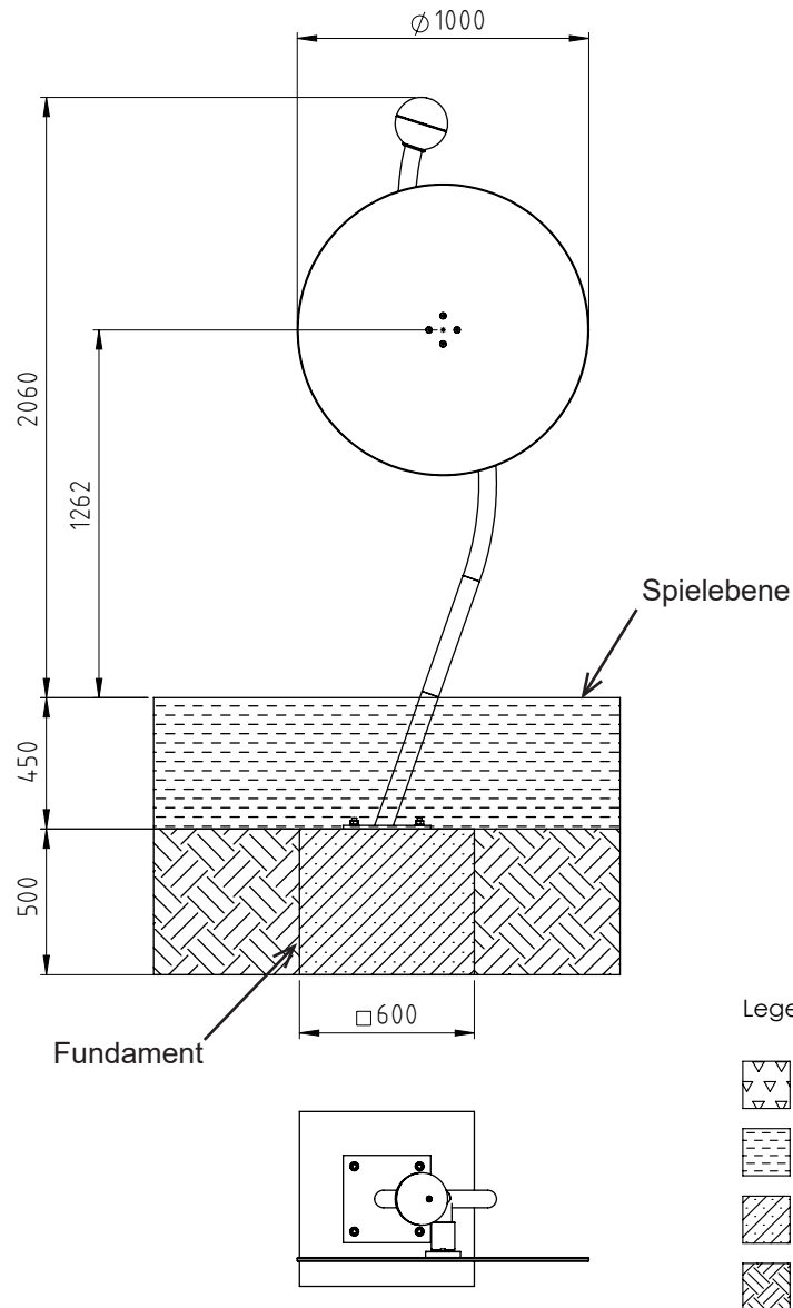
Skizze 2: Fundamentplan
