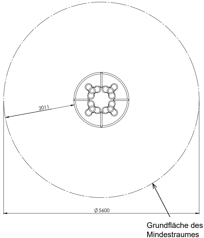
Skizze 3: Draufsicht
