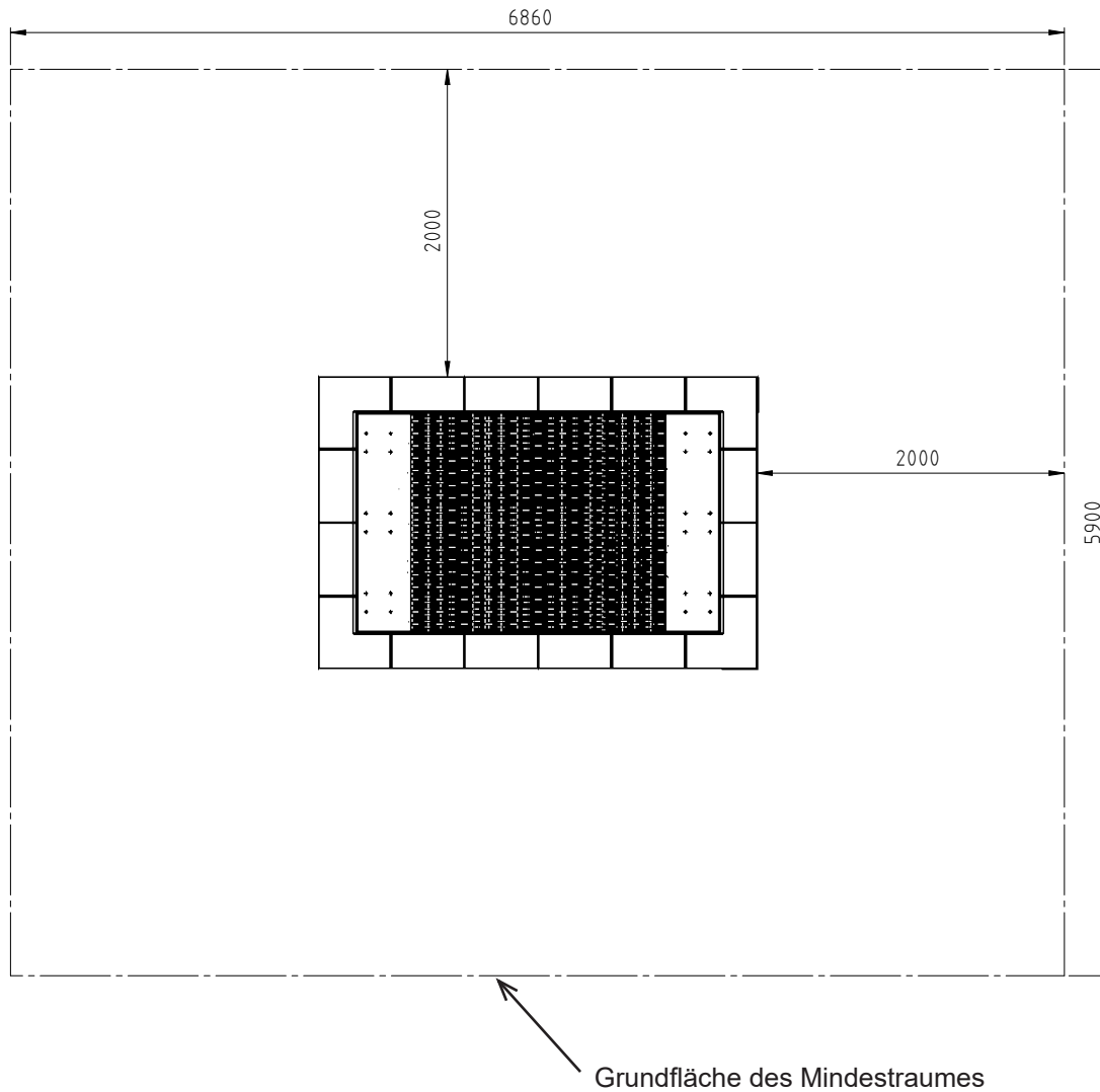
Skizze 3: Draufsicht
