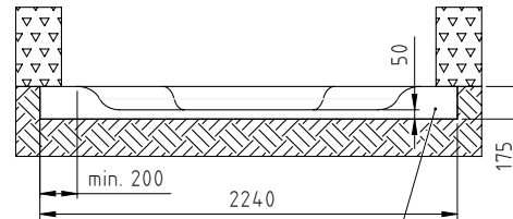
Drainageschicht drainage layer
