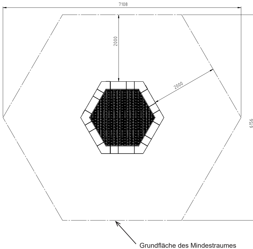
Skizze 3: Draufsicht
