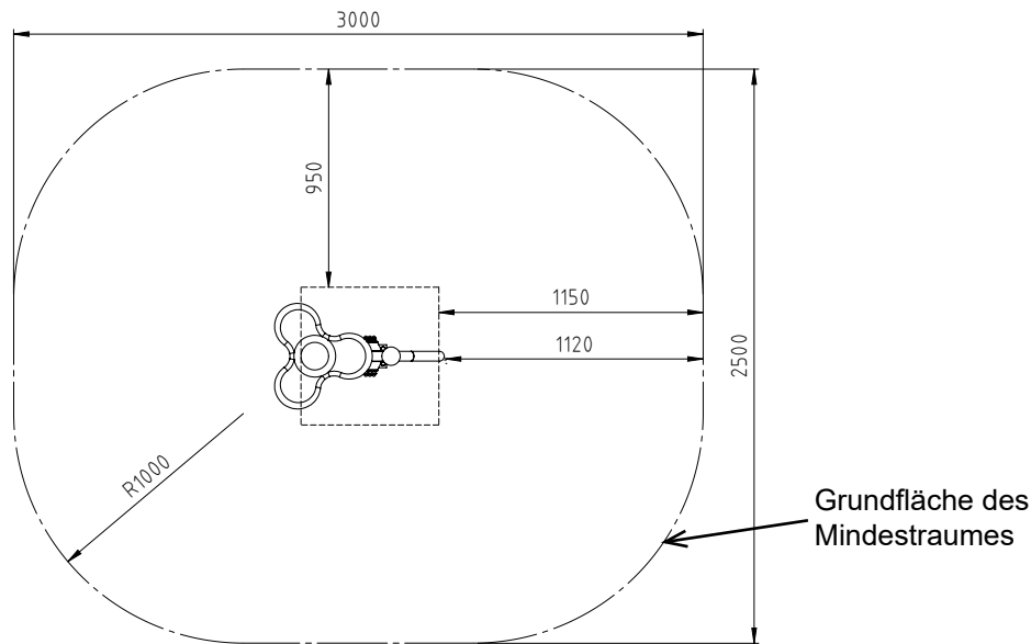
Skizze 3: Draufsicht
