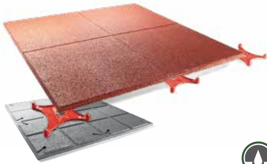
Elastikplatte 1000 x 1000 x 30 mm
