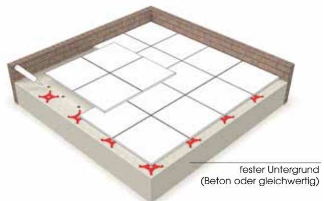
Verlegung der Elastikplatte 30 mit Hilfe des Verbindungskreuzes
