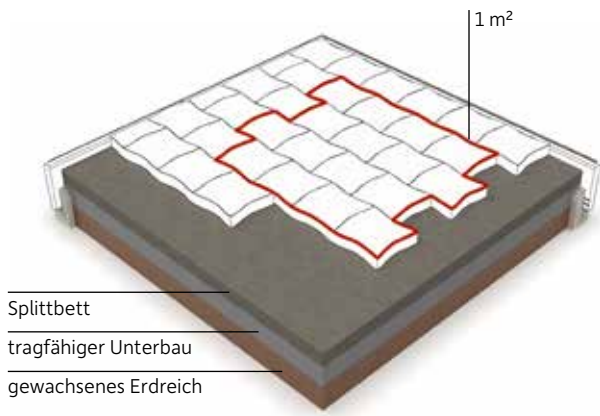
Verlegung des Terrasoft Designpflasters auf sickerfähigem Untergrund (nicht mit dem Auto befahrbar.)
