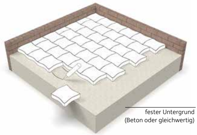
Verlegung des Terrasoft Designpflasters auf festem Untergrund
